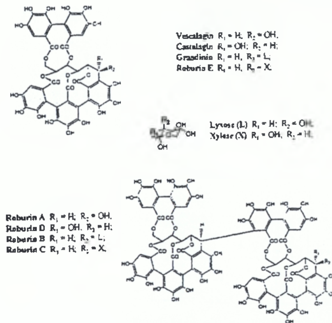
Εικόνα 8: Η δομή των 8 κυριότερων ελλαγιταννινών που έχουν ταυτοποιηθεί στο ξύλο της δρυός (Puech et al., 1999).
