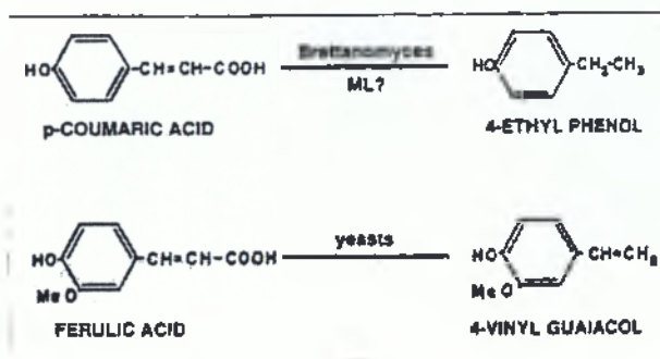
Εικόνα 16: Μετατροπή φερουλικού και κουμαρικού οξέος σε αρωματικές φαινόλες.
