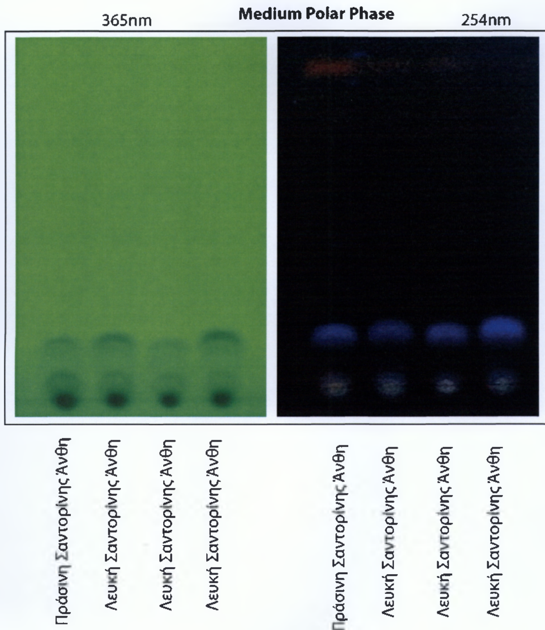
Εικόνα 2. Η ανάλυση των μεσαία πολικών ουσιών οι οποίες εκχυλίστηκαν με οξικό μεθυλεστέρα σε χρωματογραφία λεπτής στοιβάδας. Οι φωτογραφίες ελήφθησαν σε δύο διαφορετικά μήκη κύματος.
