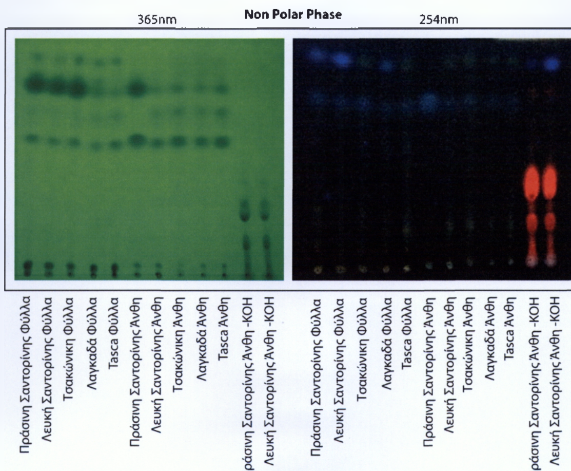
Εικόνα 1. Η ανάλυση των μη πολικών ουσιών οι οποίες εκχυλίστηκαν με εξάνιο με χρωματογραφία λεπτής στοιβάδας. Οι φωτογραφίες ελήφθησαν σε δύο διαφορετικά μήκη κύματος.
