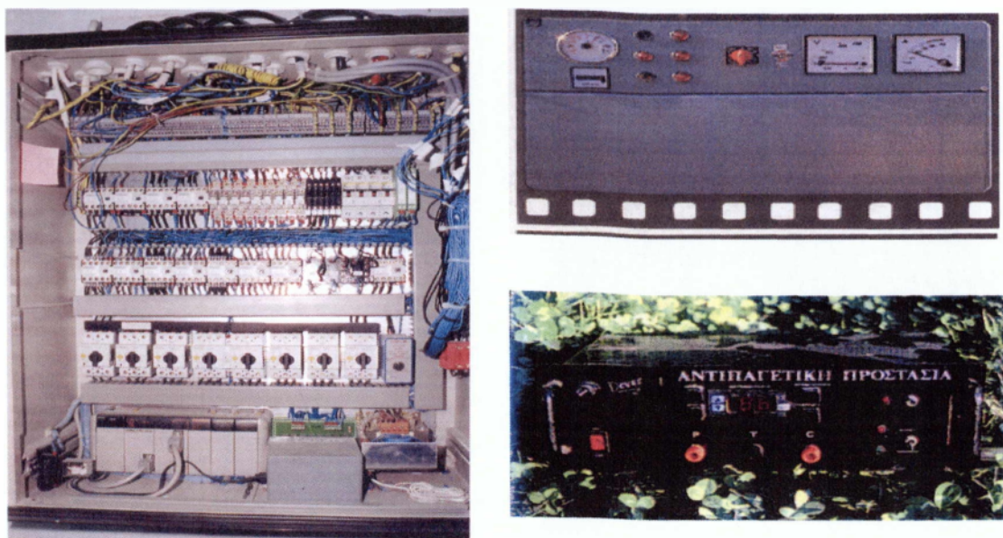
Εικόνα 9. Πίνακες συστήματος αυτοματισμού
