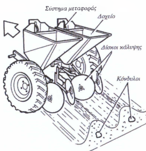
Εικόνα 3.5.Σχηματική παράσταση μηχανής φύτευσης κονδύλων
