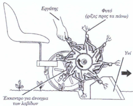
Εικόνα 3.19.Σχηματική παράσταση ημιαυτόματου μεταφυτευτικής με τροχό που φέρει λαβίδες (Ribouleau).
