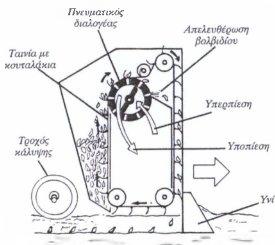
Εικόνα 3.4. Αρχή αυτόματης μηχανής φύτευσης σκόρδου (Erpe)
