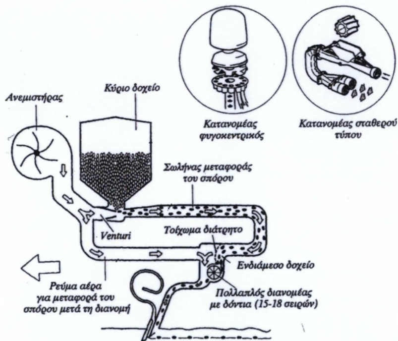
Εικόνα 2.27. Αρχή σπαρτικής γραμμικής σποράς με πολλαπλούς διανομείς και μεταφορά με ρεύμα αέρα. Κάθε διανομέας διανέμει σπόρους σε πολλές σειρές (Kongskilde)
