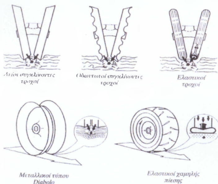
Εικόνα 2.5. Σχηματική παράσταση τροχών κάλυψης του σπόρου, μηχανών σποράς ακριβείας.
