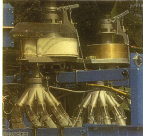
Εικόνα 2.25. Αρχές σπαρτικής γραμμικής σποράς, με πολλαπλούς ανεξάρτητους διανομείς και μεταφορά με ρεύμα αέρα
