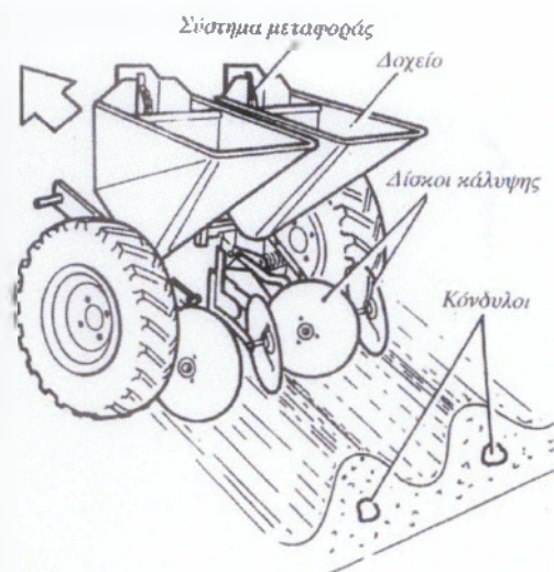
Εικόνα 3.26. Σχηματική παράσταση μηχανής φύτευσης κονδύλων
