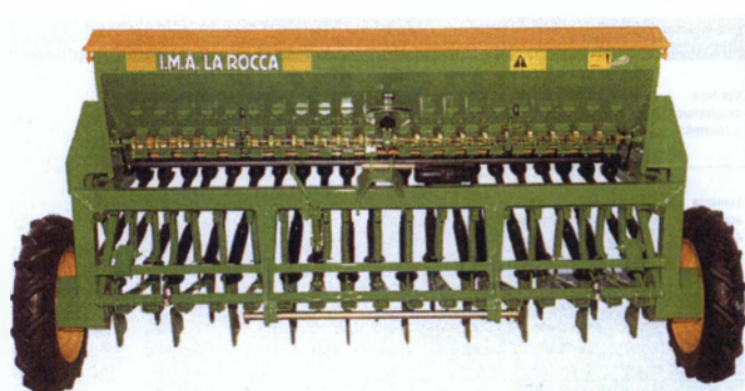
Εικόνα 2.12. Σπαρτική Μηχανή
