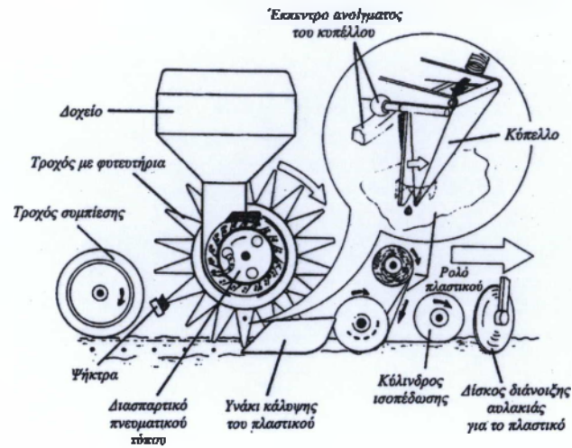
Εικόνα 1.2.Ειδική σπαρτική τύπου φυτευτηρίων με ταυτόχρονη κάλυψη πλαστικού
