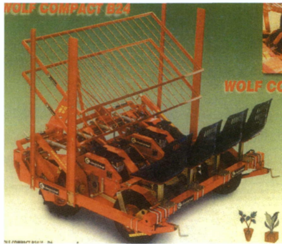
Εικόνα 3.16. Σχηματική παράσταση ημιαυτόματης μηχανής μεταφύτευσης με μεταφορική ταινία και συγκλίνοντες τροχούς (Accord)
