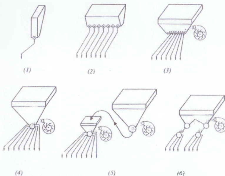
Εικόνα 2.2. Διαμόρφωση των σπαρτικών ανάλογα με το δοχείο, το διασπαρτικό σύστημα και το σύστημα μεταφοράς του σπόρου
