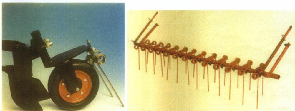
Εικόνα 2.11. Μηχανισμοί κάλυψης του σπόρου
