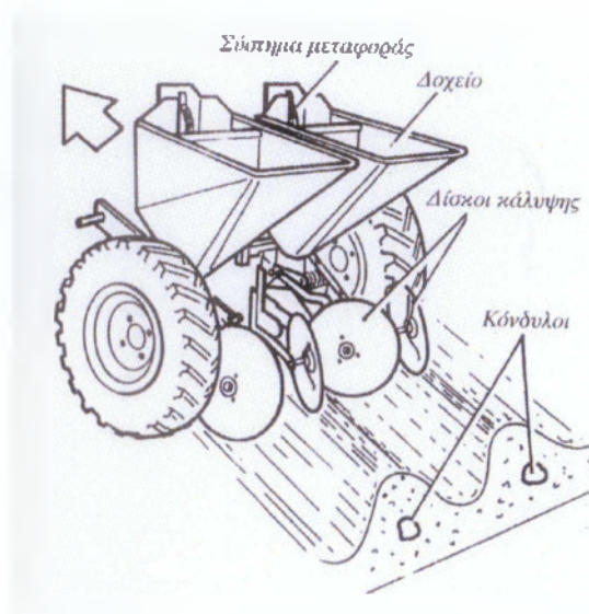
Εικόνα 3.1. Σχηματική παράσταση μηχανής φύτευσης κονδύλων
