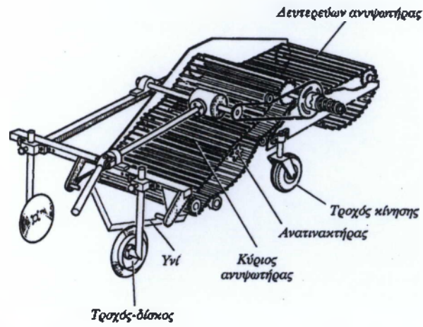
Εικόνα 1.4. Ημιφερόμενος εξαγωγέας πατάτας με ανυψωτήρα
