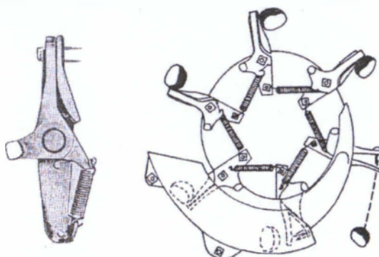
Εικόνα 3.10.Σχηματική παράσταση αυτόματης μηχανής φύτευσης κονδύλων με περιστρεφόμενο κατακόρυφο τροχό με βραχίονες που φέρουν βελόνα αγκίστρωσης. Αριστερά μηχανισμός αγκίστρωσης
