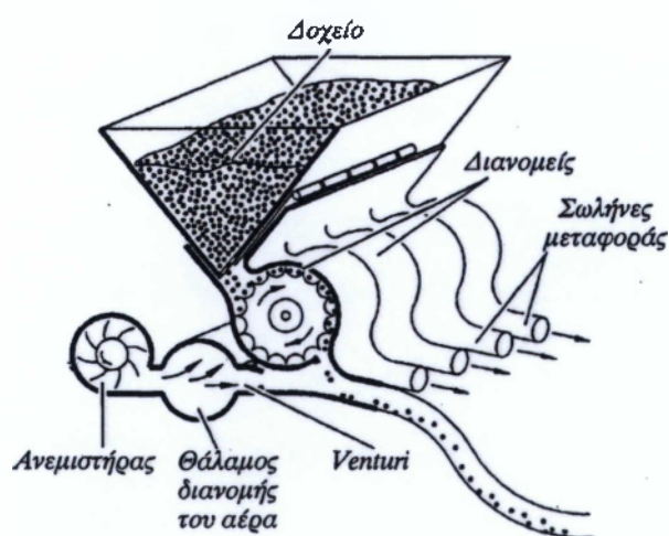
Εικόνα 2.16. Περιγραφή δοχείου σπαρτικής μηχανής
