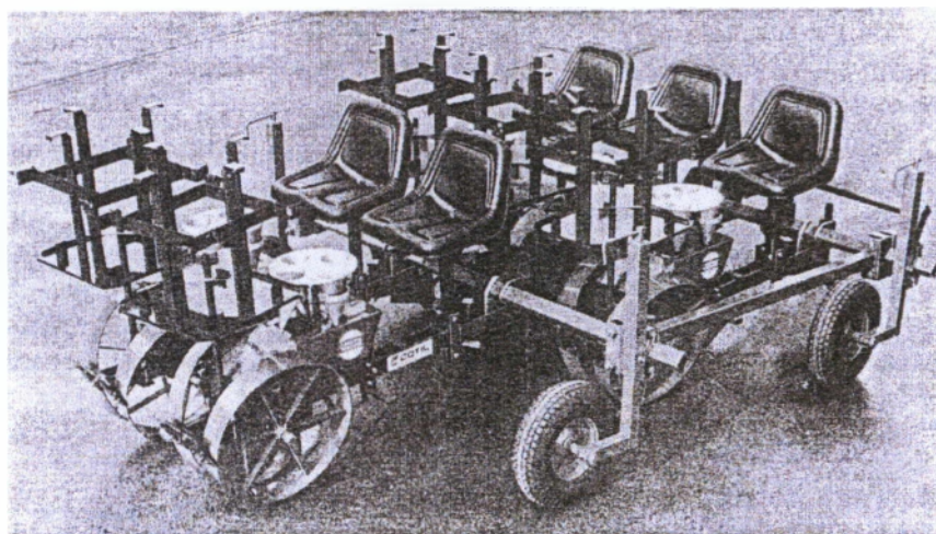
Εικόνα 3.23. Ημιαυτόματη μηχανή 5 σειρών για μεταφύτευση φυτών με μπάλα χώματος (A και B αρχές λειτουργίας)
