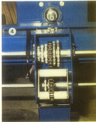
Εικόνα 2.22. Κιβώτια μετάδοσης της κίνησης σε μηχανές γραμμικής σποράς
