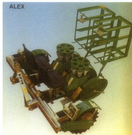
Εικόνα 3.17. Ημιαυτόματη μεταφύτευτική με μεταφορική ταινία που φέρει λαβίδες (Colchester tillage)
