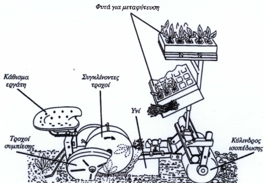
Εικόνα 2.4. Σχηματική παράσταση ημιαυτόματης μηχανής μεταφύτευσης με συγκλίνοντες ελαστικούς τροχούς (Accord)
