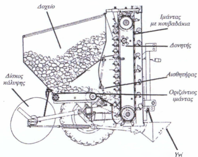
Εικόνα 3.8.Αυτόματη μηχανή φύτευσης κονδύλων με κουβαδάκια
