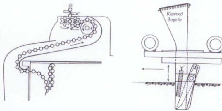
Εικόνα 3.25. Αρχές αυτόματης μηχανής μεταφύτευσης, με συνεχή τροφοδότηση των φυτών (Hauser, V. L. 1985)
