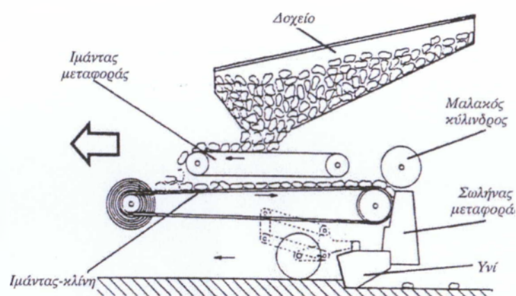
Εικόνα 3.9.Σχηματική παράσταση μηχανής φύτευσης με ιμάντες (Gregoire et Besson)
