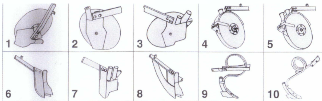
Εικόνα 2.24. Σώματα διάνοιξης της αυλακιάς, κλασικής μηχανής γραμμικής σποράς
