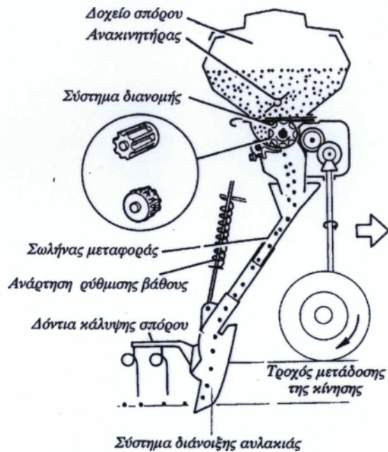
Εικόνα 1.3. Σύστημα διάνοιξης αυλακιάς
