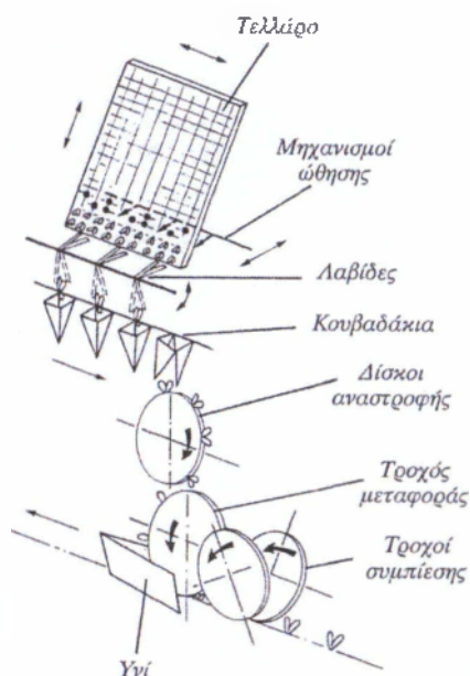
Εικόνα 3.24. Αρχές αυτόματης μηχανής μεταφύτευσης (Simon)
