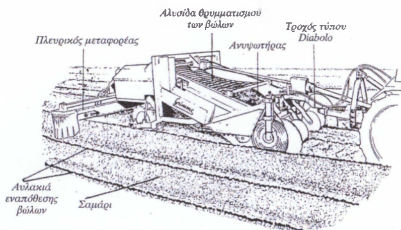
Εικόνα 3.3.Ειδικό μηχανήμα που απομακρύνει πέτρες και βόλους από το έδαφος πριν από τη φύτευση της πατάτας. Οι βόλοι εναποτίθενται στην παρακείμενη αυλακιά (Grimme)
