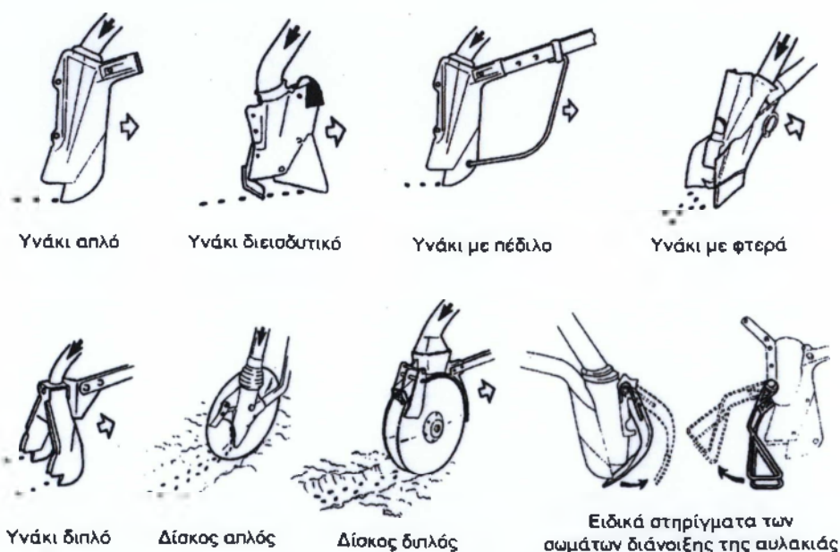
Εικόνα 2.23. Σώματα διάνοιξης της αυλακιάς, κλασσικής μηχανής σποράς
