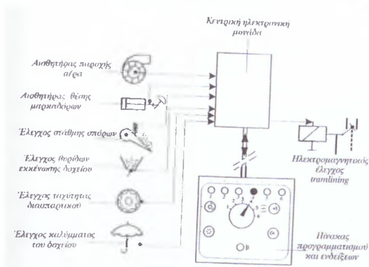
Εικόνα 2.9. Σχηματική παράσταση κυκλωμάτων αυτοματισμού μιας σύγχρονης σπαρτικής
