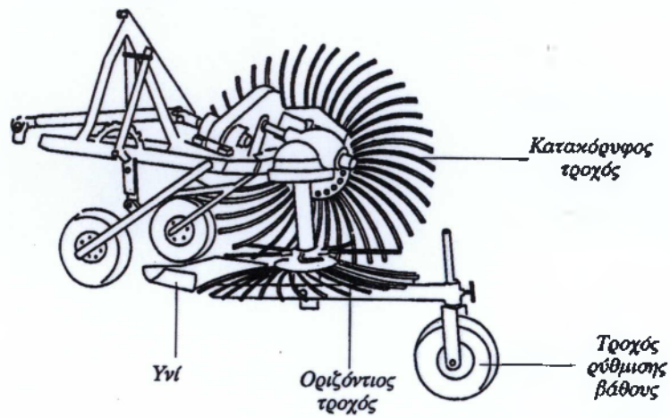
Εικόνα 1.5. Εξαγωγέας πατάτας με δύο περιστρεφόμενους τροχούς με δόντια
