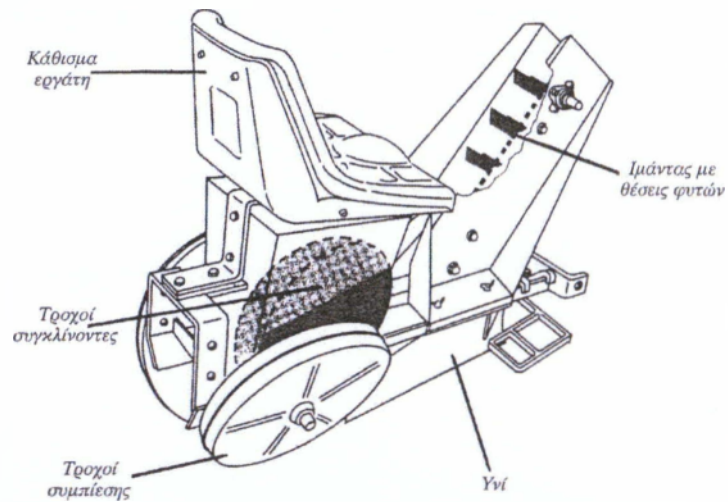
Εικόνα 3.18.Σχηματική παράσταση ημιαυτόματης μηχανής μεταφύτευσης με μεταφορική ταινία για συγκλίνοντες τροχούς (Accord)
