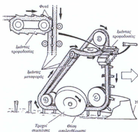
Εικόνα 3.22. Σχηματική παράσταση ημιαυτόματης μεταφύτευτικής με ιμάντες (Gregoire et Besson)
