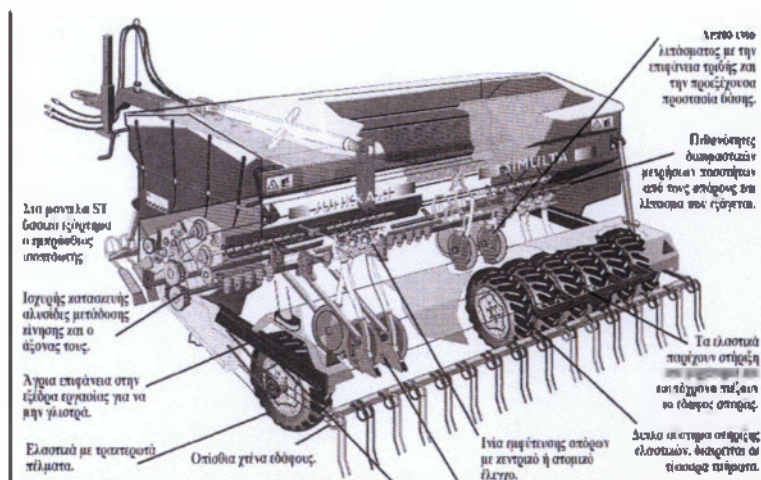
Εικόνα 2.13. Περιγραφή Σπαρτικής Μηχανής
