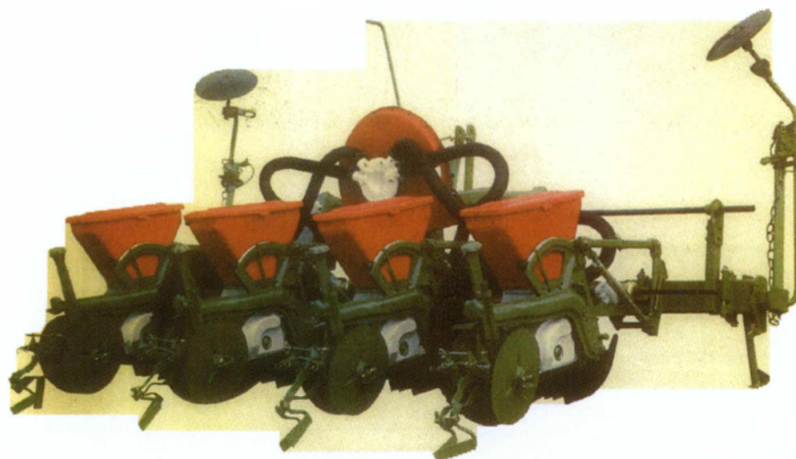
Εικόνα 2.31. Πνευματική σπαρτική ακριβείας.
