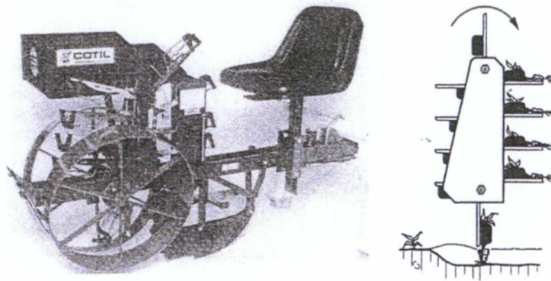
Εικόνα 3.20. Ημιαυτόματη μεταφυτευτική με μεταφορική ταινία που φέρει λαβίδες (Colchester tillage)
