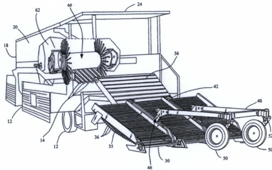
Εικόνα 3.12. Μεταφυτευτική μηχανή πατάτας
