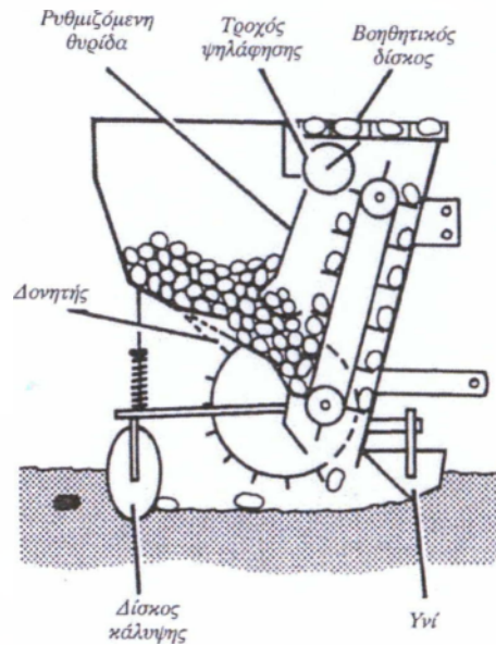
Εικόνα 3.7. Ημιαντόματο σύστημα φύτευσης κονδύλων
