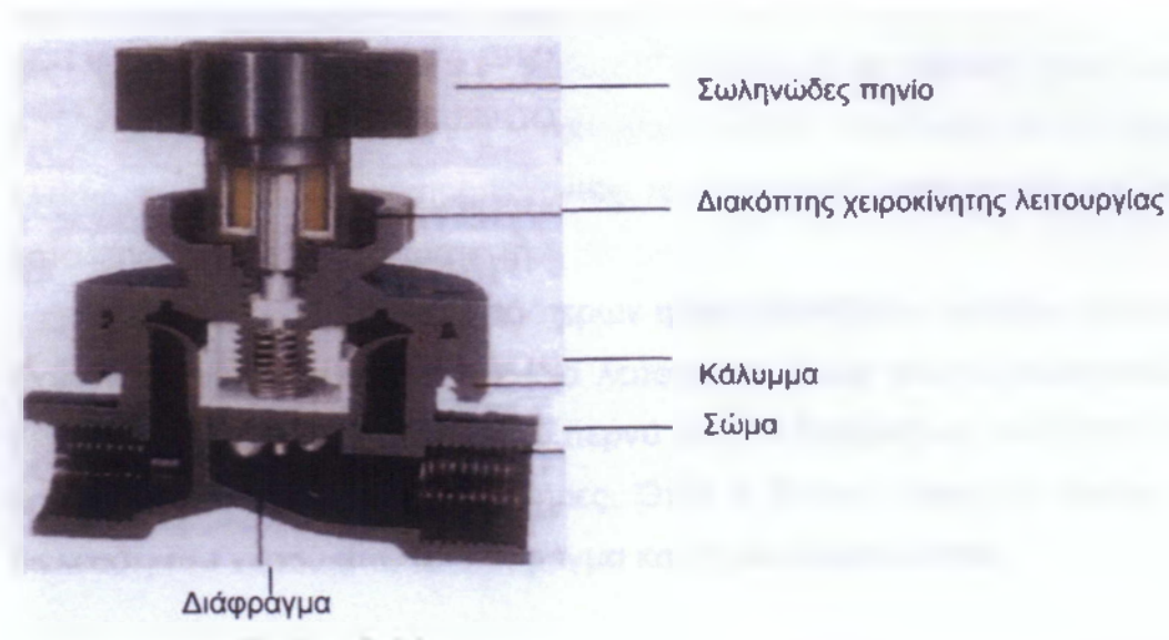
Εικόνα 3.14 Ηλεκτροβαλβίδα σε τομή
